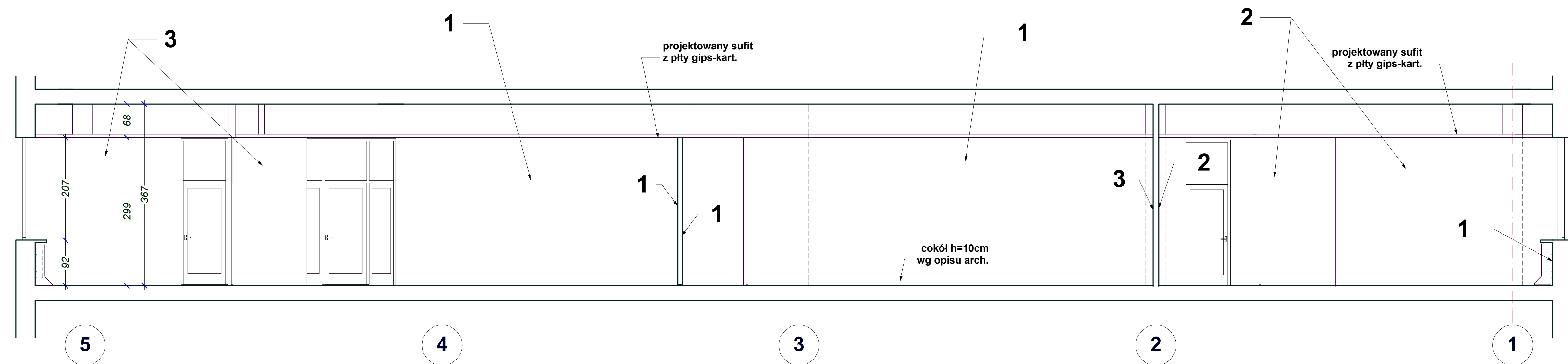
WIDOK C-C
