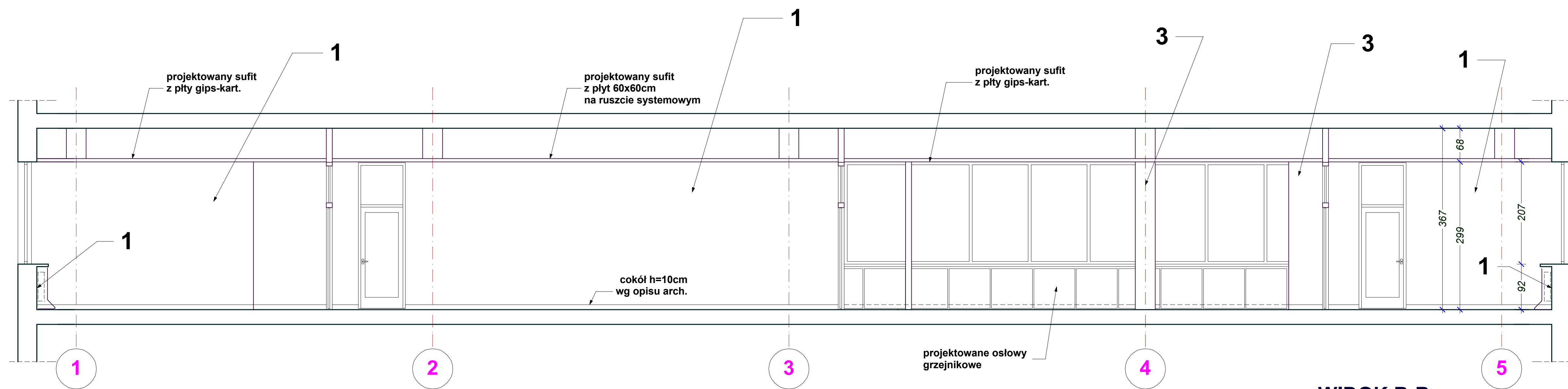
WIDOK B-B
